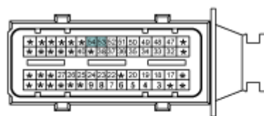
TCM 连接器 [CHG-A]
