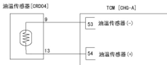
[电路图]
